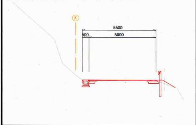
計画横断面図（案） ①-①（待避所）
