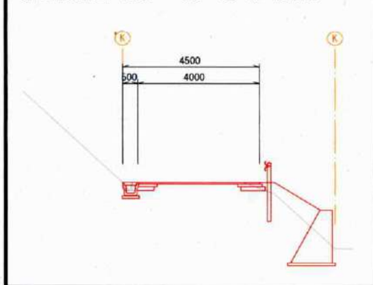
計画横断面図（案） ②-②（一般部）
